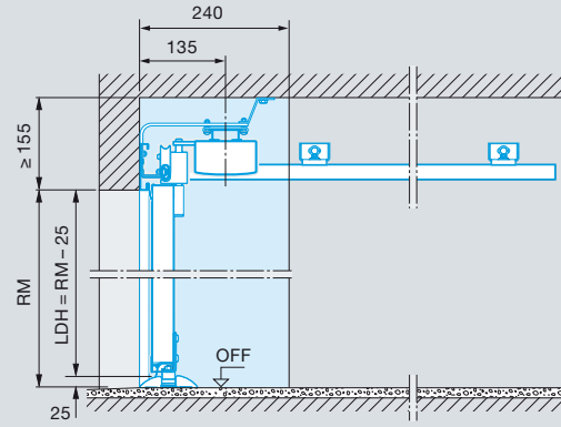
ES-Beschlag (Einfachschiene) Antrieb Deckenmontage A
