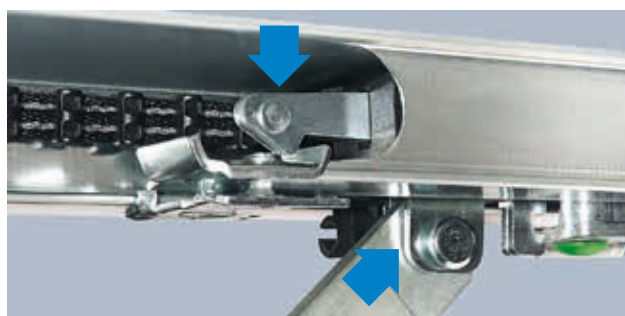
Torverriegelung über die Antriebsschiene (Europäisches Patent)
