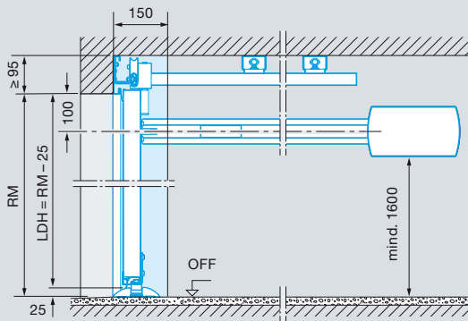
ES-Beschlag (Einfachschiene) Antrieb Wandmontage
